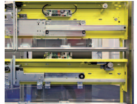
Türantrieb im Standby stromlos
